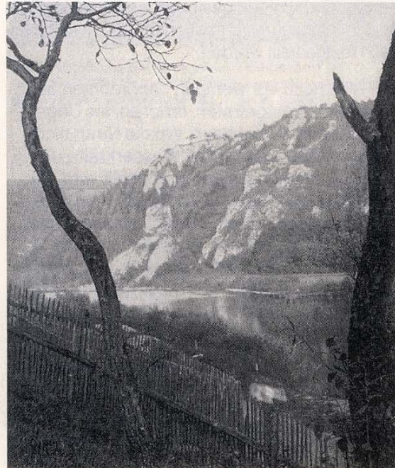
Drabafelsen bei Etterzhausen (Oberpfalz)
